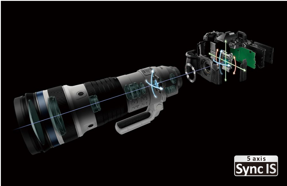
[ボディ内の5軸手ぶれ補正機構]と[レンズ内の手ぶれ補正機構]を協調させることにより、超望遠撮影における補正効果を最大化
