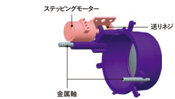
ステッピングモーターを利用したMSC機構
