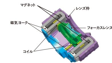
VCM(Voice Coil Motor)を利用したMSC機構
