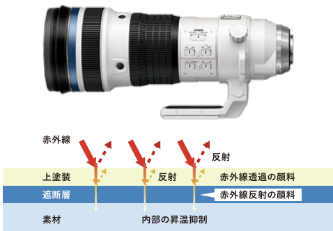
太陽光下でも温度上昇を抑える遮熱白塗装
